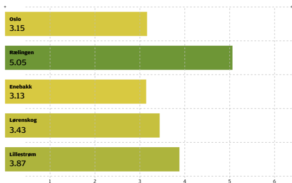
VA13 Antall stopp i kloakken per 100 km spillvannsnett
